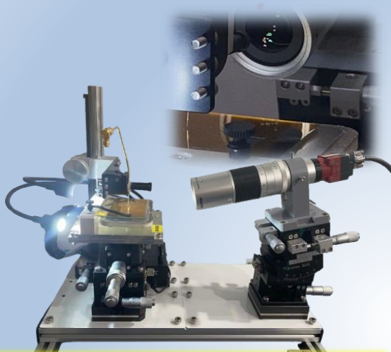
硬化・乾燥過程のリアルタイムモニタリング 電場ピックアップシステム
